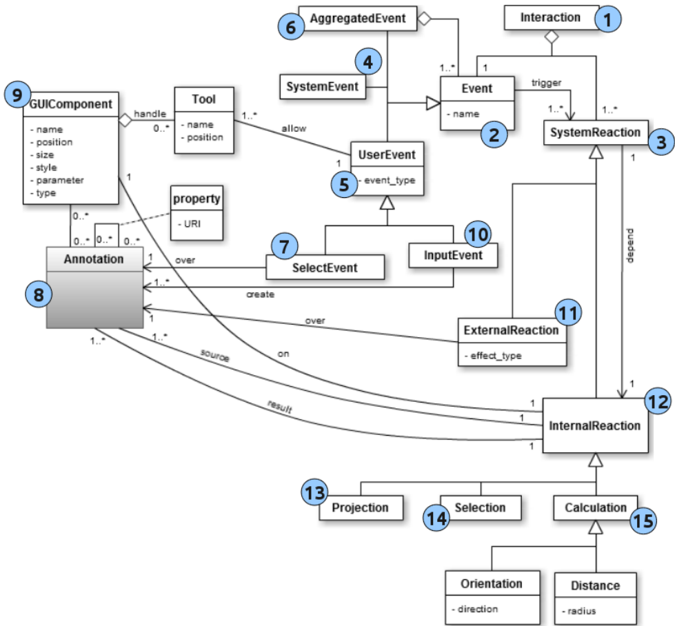
Fig. 12. Modèle de description des interactions
