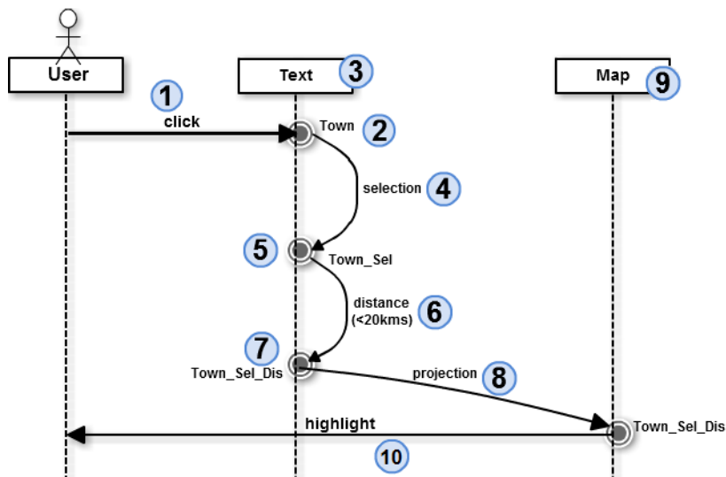
Fig. 19. Exemple d'un diagramme d'interaction
