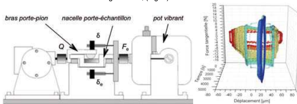
Fig. 1 (a) Dispositif de fretting à déplacements libres : position des capteurs de force et de déplacement en entrée ( F_e , \delta_e ) et en sortie ( Q , \delta ) du contact, (b) évolution des cycles de fretting au cours d'un essai conduisant au grippage : lorsque l'effort tangenciel croît, le débattement se réduit.
