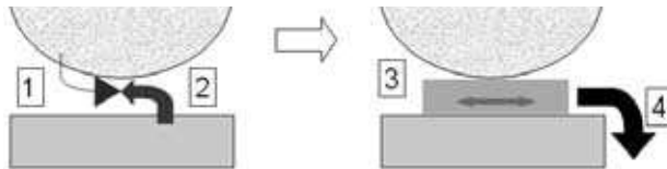
Fig. 9 Scénario d'usure et débits de matière dans le cas du composite 4%NTC-7%Fe- \text{Al}_2\text{O}_3 face à un frotteur en alumine 99,7% FN (même symbolisme que la figure 9).
