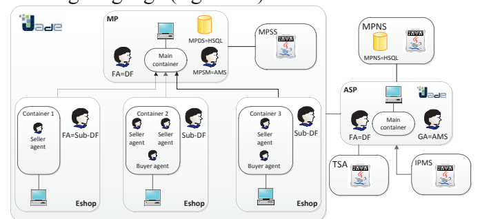
Fig. 13. The MP-Jade framework
