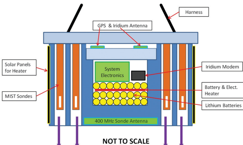
FIG. 3. Driftsonde gondola.
