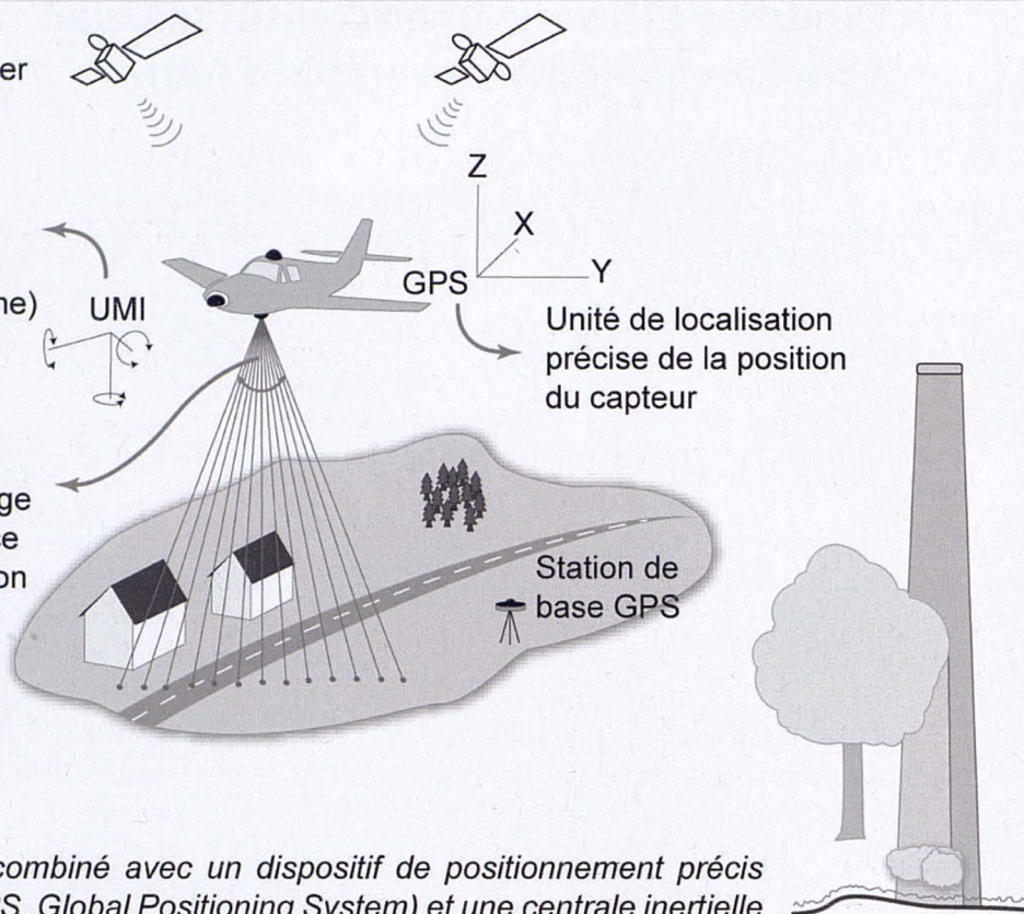
Fig. 1 Principe du système laser aéroporté LIDAR ( Light Détection and Ranging ), (d'après Ž. Kokalj et K. Oštir, in, Rodier et al., 2011)
