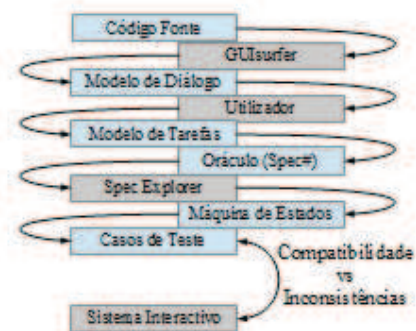
Figura 2: Geração de casos de teste baseado em modelos
