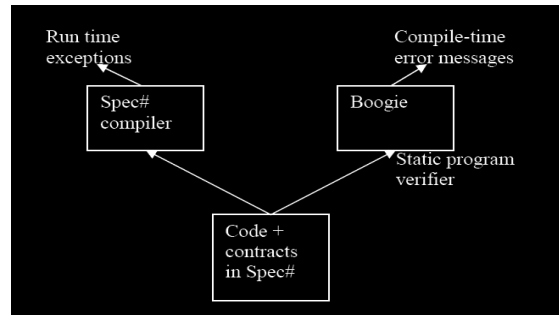
Figura 1: O sistema de programação Spec#
