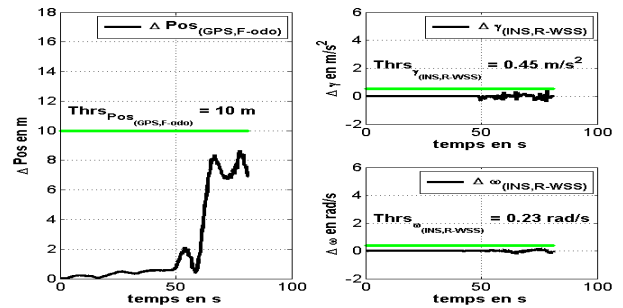
FIGURE 16. Faute logicielle dans KF_2 : Comparaison des capteurs
