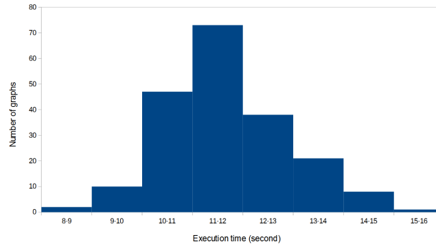
FIG. 6 – Histogramme des temps d'exécution de l'algorithme principal
