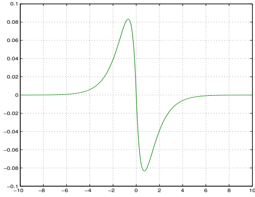
(b) \rho'(x) = (\frac{1}{3}e^{-|x|} - \frac{1}{3}e^{-2|x|})_{x<0} + (\frac{1}{3}e^{-2|x|} - \frac{1}{3}e^{-|x|})_{x>0} profile.
