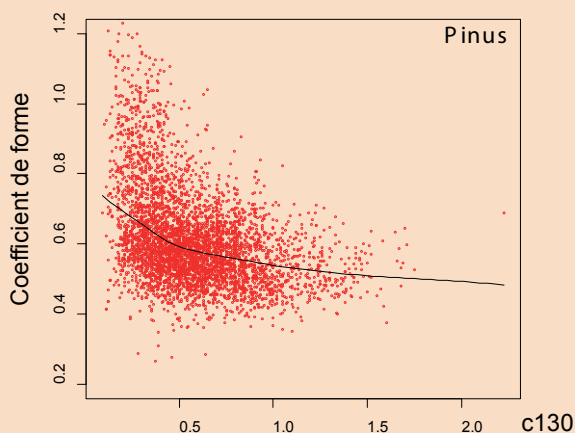
Fig. b : représentation du coefficient de forme formTot (tige et branches), calculé pour les pins, en fonction de la taille des arbres (circonférence à 1,30 m)
