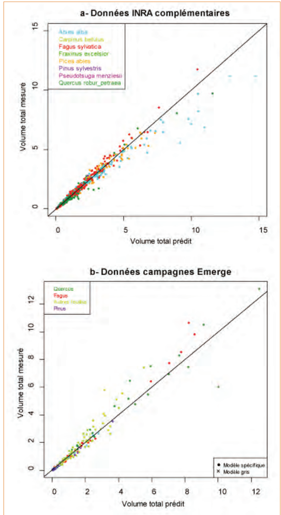
Fig. 2 : tests du modèle de volume total sur deux jeux de données indépendantes : en haut, des données INRA n'ayant pas servi à la phase de calibration; en bas, celles des 226 arbres mesurés pendant le projet. Les prédictions, en abscisses, sont comparées aux volumes mesurés, en ordonnées. La droite correspond à l'égalité entre valeur prédite et valeur mesurée.
