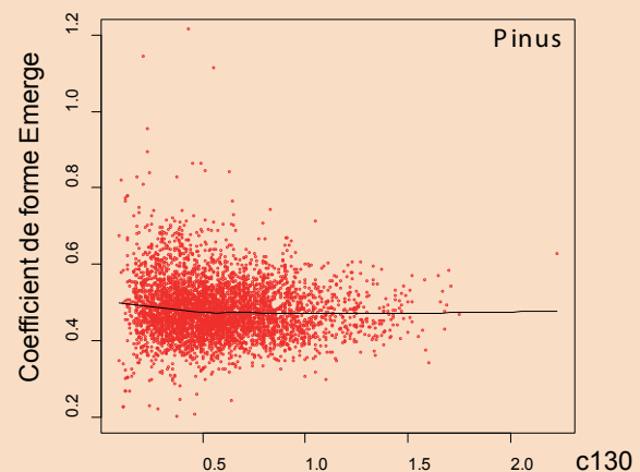
Fig. d : représentation du coefficient corrigé formTotNew , calculé pour les pins, en fonction de la taille des arbres (circonférence à 1,30 m).
