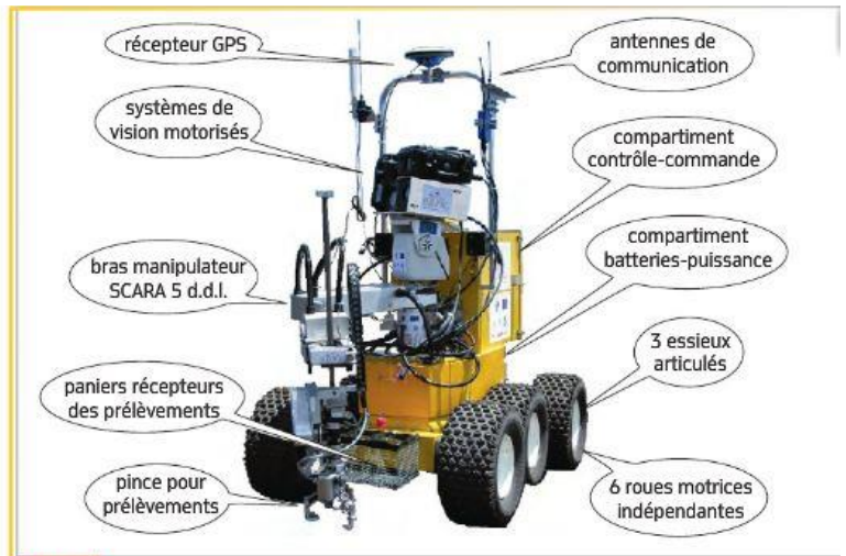
Fig. 2 Principaux constituants
