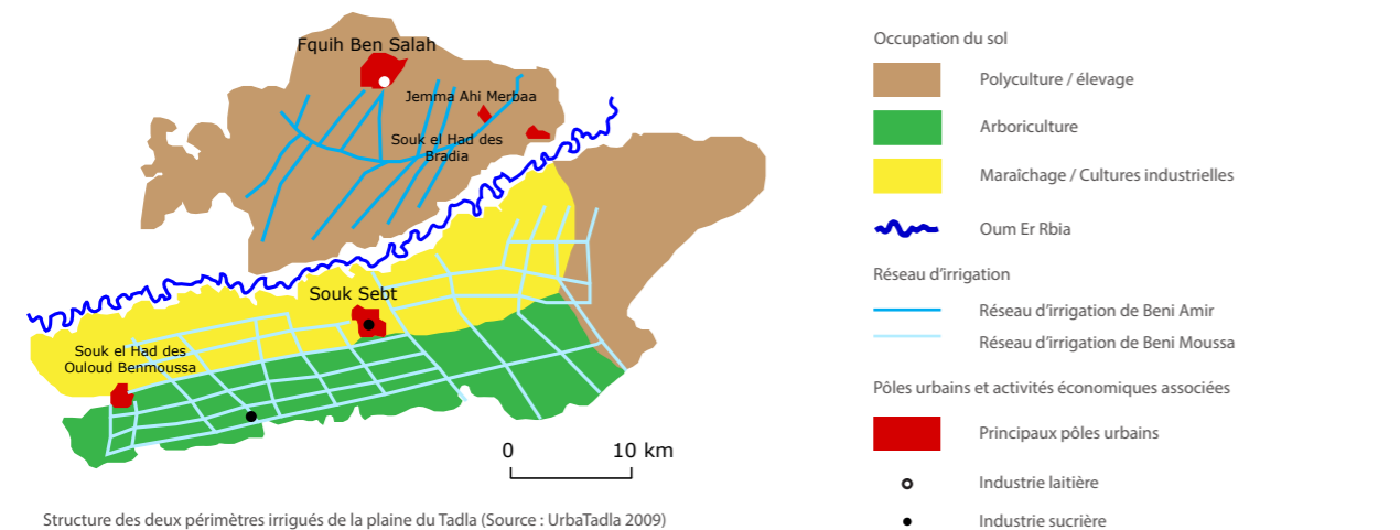
Structure des deux périmètres irrigués de la plaine du Tadla (Source : UrbaTadla 2009)
