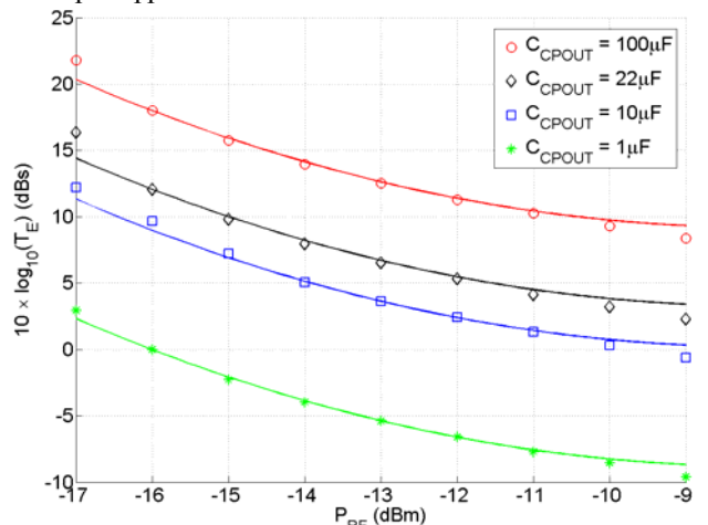
Figure 7. Mesure et caractérisation de T_E en fonction de la puissance P_{RF} en entrée du redresseur.
