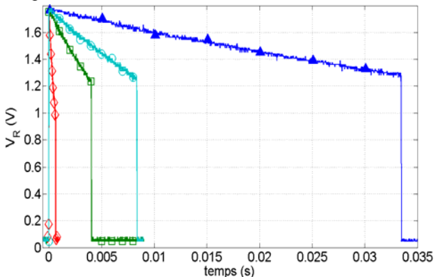
Figure 6. Mesure de la tension en sortie du circuit de pompe de charge sur une résistance de 1kΩ pour quatre valeurs de capacités C_{CPOUT} . (▲) C_{CPOUT} = 100\mu F , (□) C_{CPOUT} = 22\mu F , (○) C_{CPOUT} = 10\mu F , et (◇) C_{CPOUT} = 1\mu F
