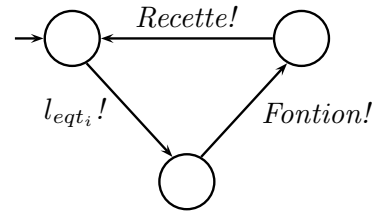
FIGURE 6. Modèle générique d'automate générateur d'événements
