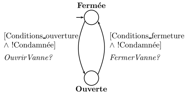
FIGURE 3. Modèle générique du comportement d'une vanne
