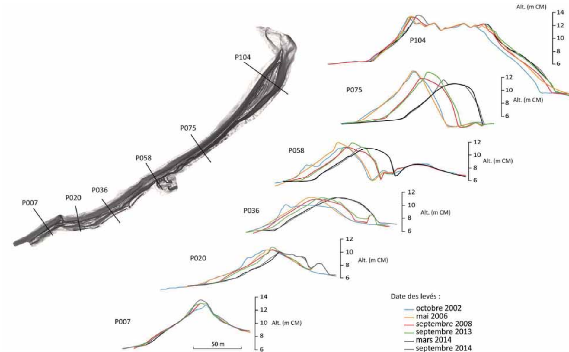
Figure 8 : Evolution morphologique du Sillon de Talbert le long de quelques profils caractéristiques.
