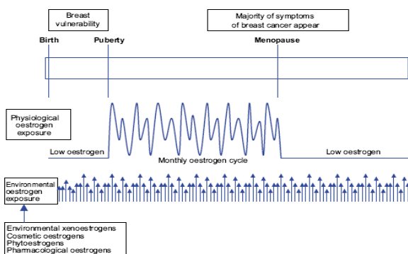
Figure 3 : Importance potentielle de la période d'exposition à des perturbateurs endocriniens environnementaux : les taux d'oestrogènes endogènes chez la femme sont élevés de la puberté à la ménopause et présentent des pics pendant les cycles menstruels qui rendent négligeables les variations apportées par l'exposition environnementale (11)
