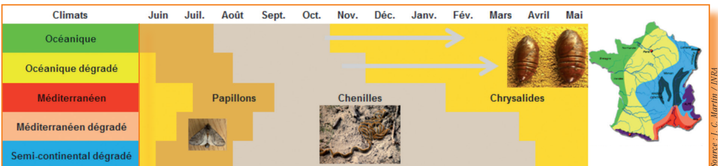
figure 2 : Présentation de la mise en correspondance du type de climat avec le cycle de vie de la processionnaire du pin. Les flèches indiquent la durée potentielle de la phase larvaire.
