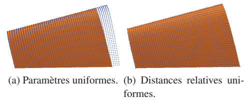
Figure 5: Deux méthodes d'échantillonnage d'une face de BRep.
