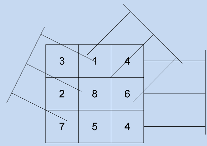
Acquisition Radon : non uniformité de la contribution des pixels dans les projections car l'échantillonnage radial et angulaire est constant.
