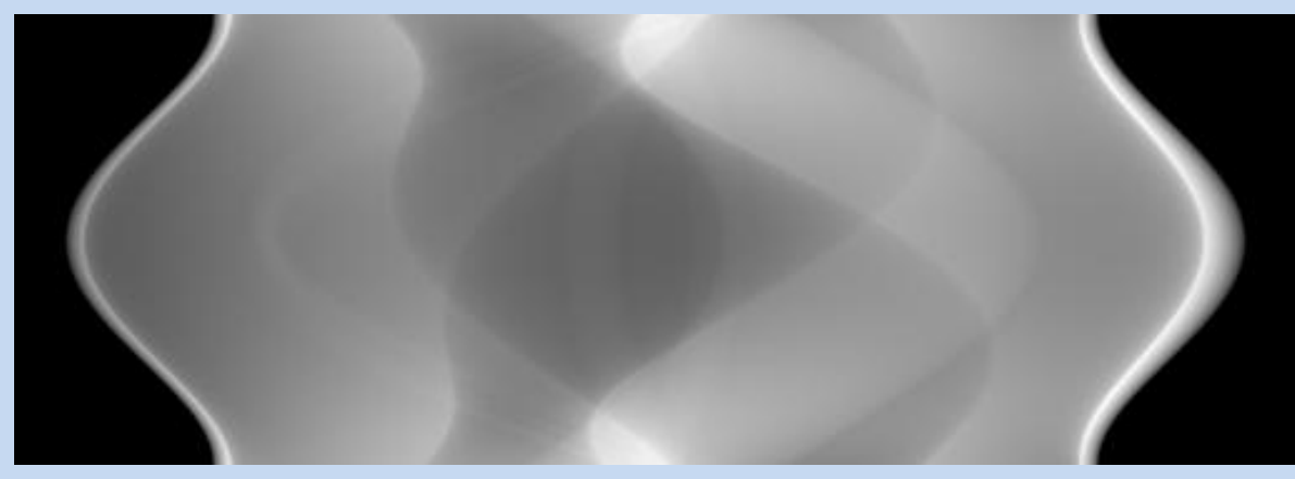
Sinogramme de Radon du fantôme d'acquisition 180 angles uniformément réparties entre 0° et 179° par pas de 1° (en colonne) de 512 échantillons par projection (en ligne).
