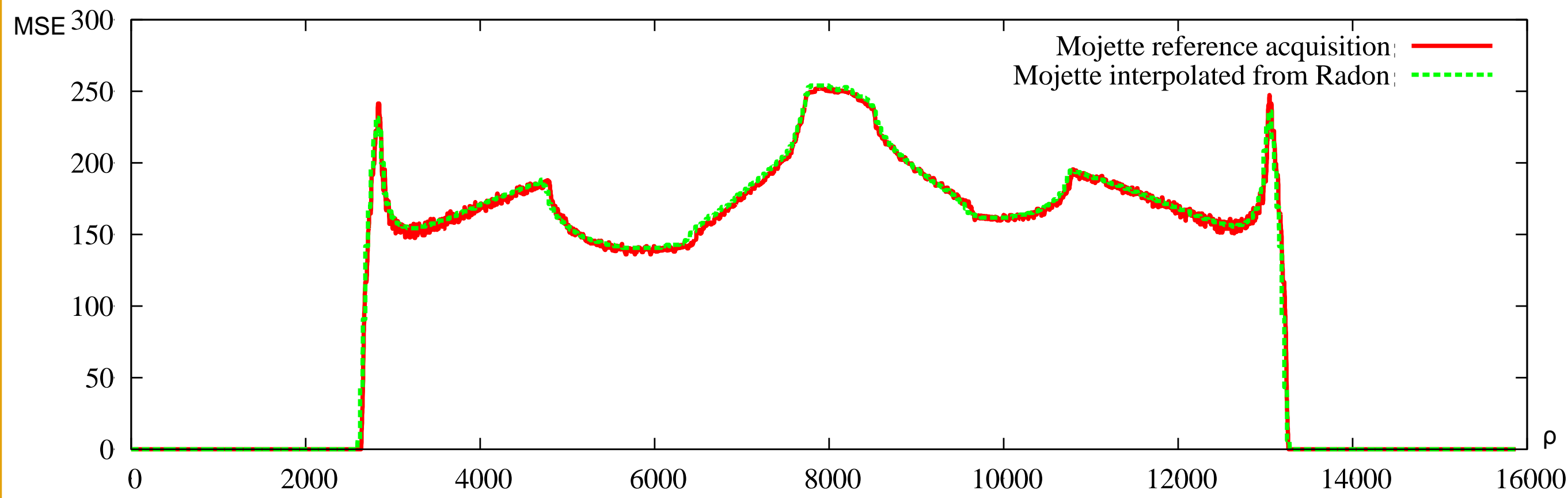
Comparaison des profils entre une projection Mojette interpolée depuis le sinogramme de Radon et la projection Mojette correspondante, acquise depuis le fantôme de Shepp-Logan.
