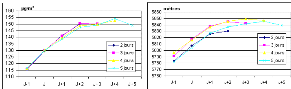
Figure 2 : Comportement moyen de l'ozone dans l'ensemble du réseau en fonction de la durée de l'épisode de pollution par l'ozone entre 1998 et 2009 dans les Alpes-Maritimes (à gauche). Evolution de l'altitude de la surface 500 hPa au dessus des Alpes-Maritimes pendant une séquence de jours pollués par l'ozone entre 1998 et 2009 (à droite).
