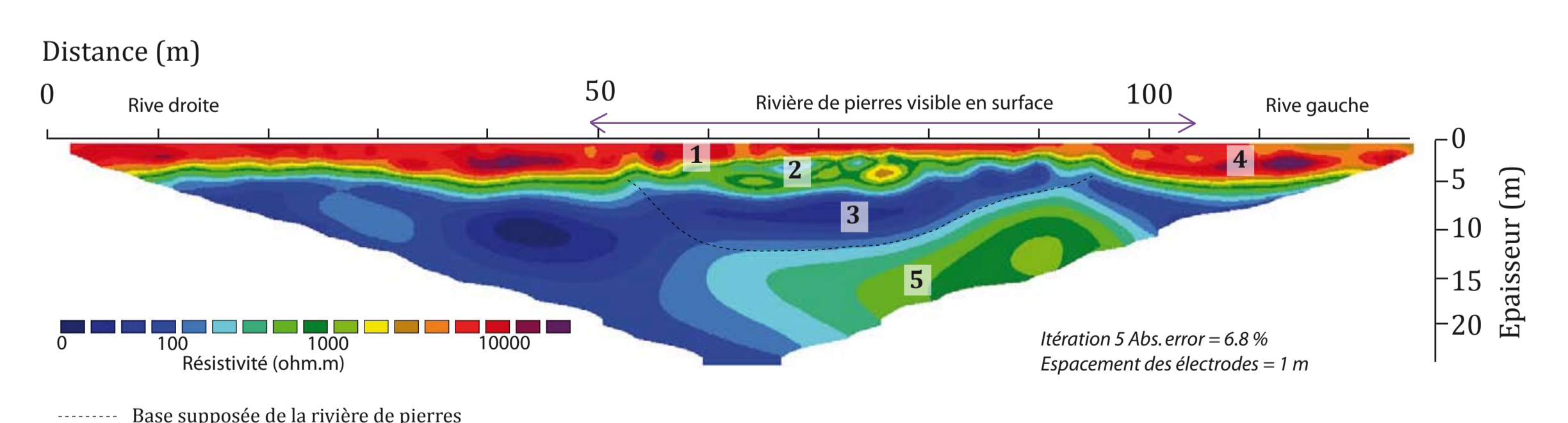
Profil GPR Pré-du-bois bas Profil de résistivité
