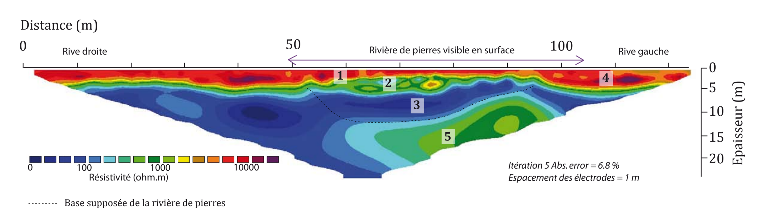
Profil GPR Pré-du-bois bas Profil de résistivité
