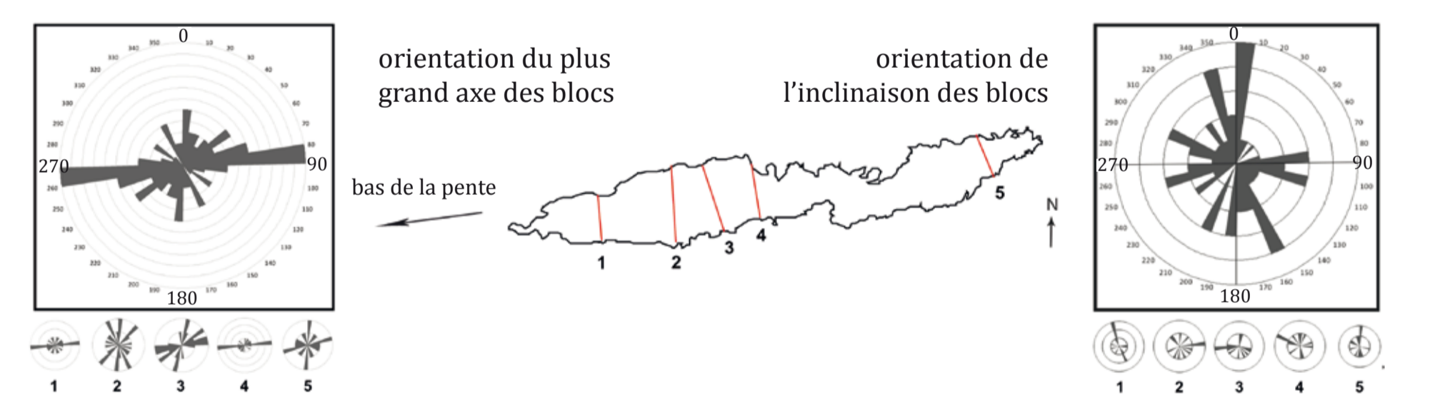
Pré-du-bois bas : étude de fabrication. Mesures effectuées sur le terrain à raison de 5 transects par rivière de pierres et 12 blocs mesurés par transect (donc 60 échantillons)
