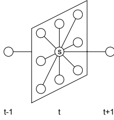
Fig. 1 spatiotemporal topology
