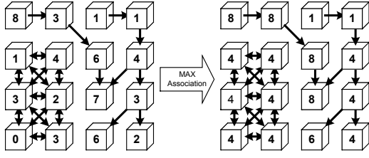
Fig. 8 MAX-Association
