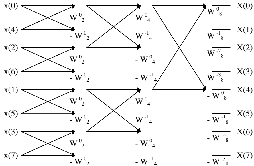
57. Graphe de fluence de la TFD rapide d'ordre 8
