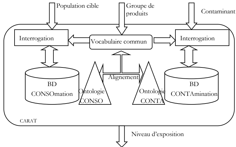
Figure 1 : Architecture du système d'intégration de données du logiciel CARAT
