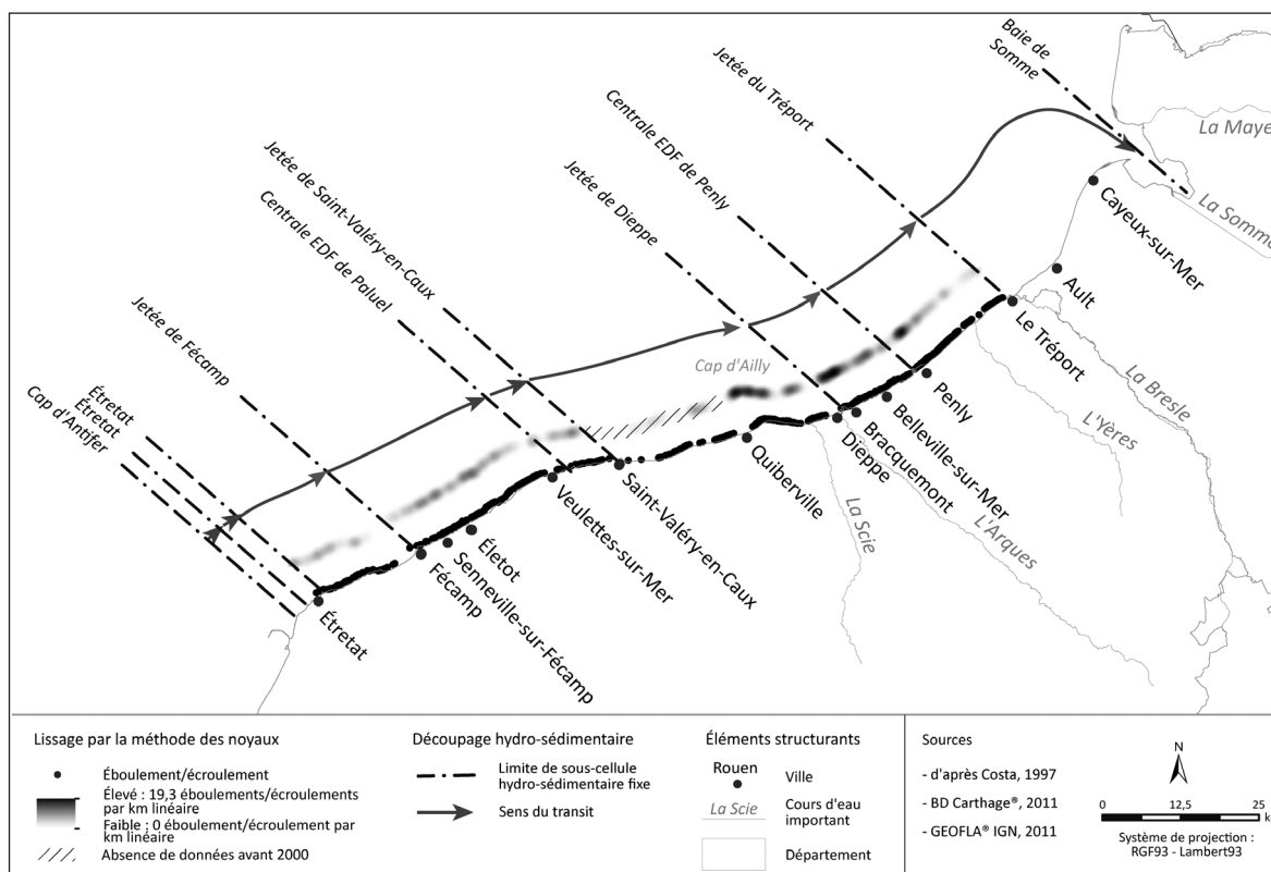
Fig. 6 – Densité (lissage par la méthode des noyaux) du nombre d'éboulements/écroulements recensés (par km linéaire) entre Étretat et Le Tréport (1939-2008). Fig. 6 – Density (kernel) of falls number censed (per linear km) from Etretat to Le Tréport (1939-2008).
