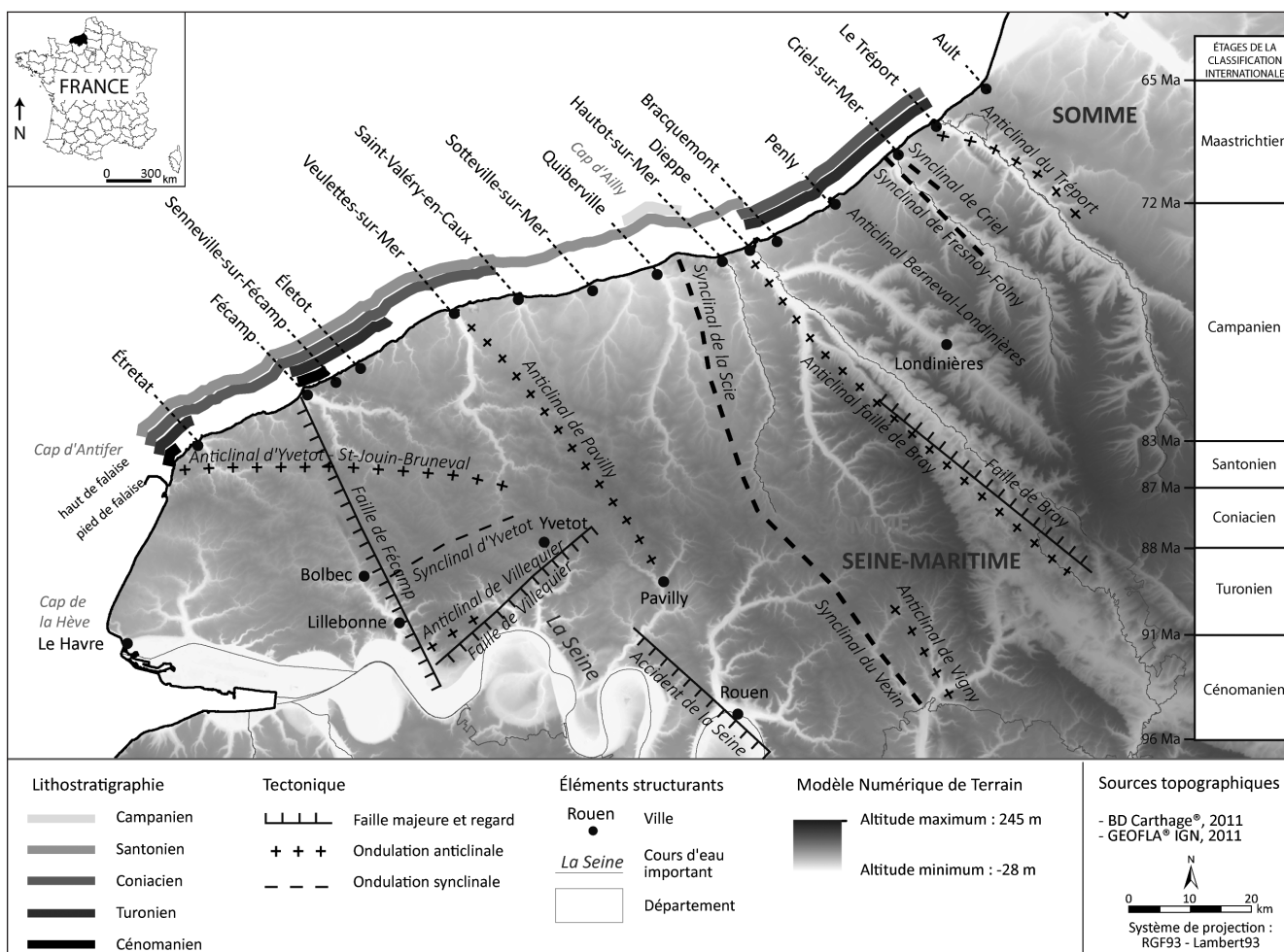
Fig. 1 – Schéma structural et lithostratigraphie simplifiée en Haute-Normandie (d'après Mégnyen et Mégnyen, 1980 in Costa, 1997 ; Laignel, 1997).
