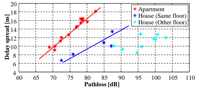
Fig. 15. Delay spread parameter versus path loss parameter
