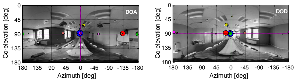
(d) Spatial distribution of deterministic paths
