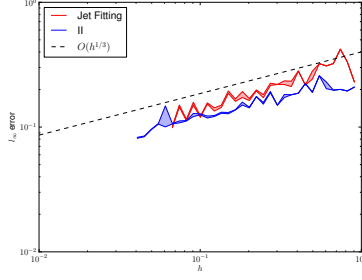
(b) RoundedCube- \hat{H}_R-l_\infty
