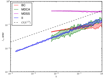
(d) Ellipse- \hat{\kappa}_R - l_\infty
