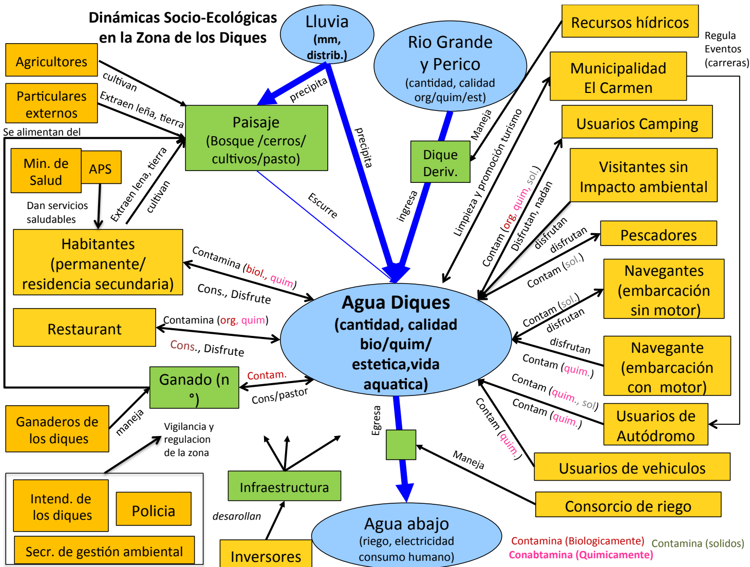
Ilustración 16: Modelo PARDI de las Dinámicas Socio-Ecológicas en la Zona del los Diques
