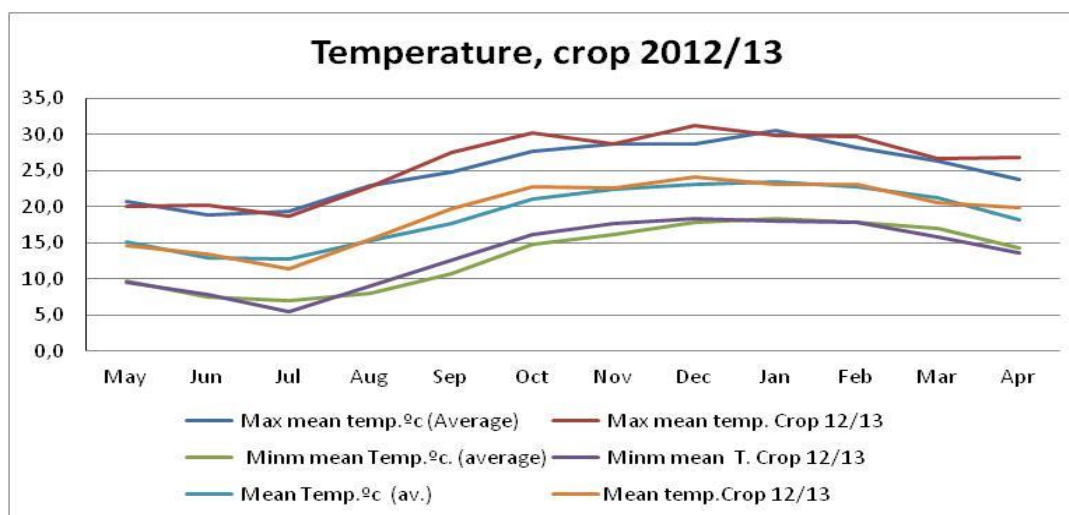
Ilustración 8: Temperaturas (promedias máx. y mín. en 15 años; promedia en 2012/2013)
