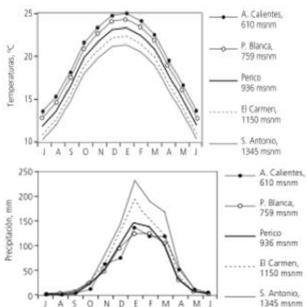
Ilustración 6: Temperaturas y precipitaciones promedio en las principales localidades
