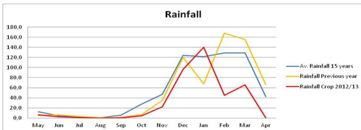
Ilustración 7: Precipitaciones mensuales en promedio sobre 15 años, en 2011/2012 y 2012/2013
