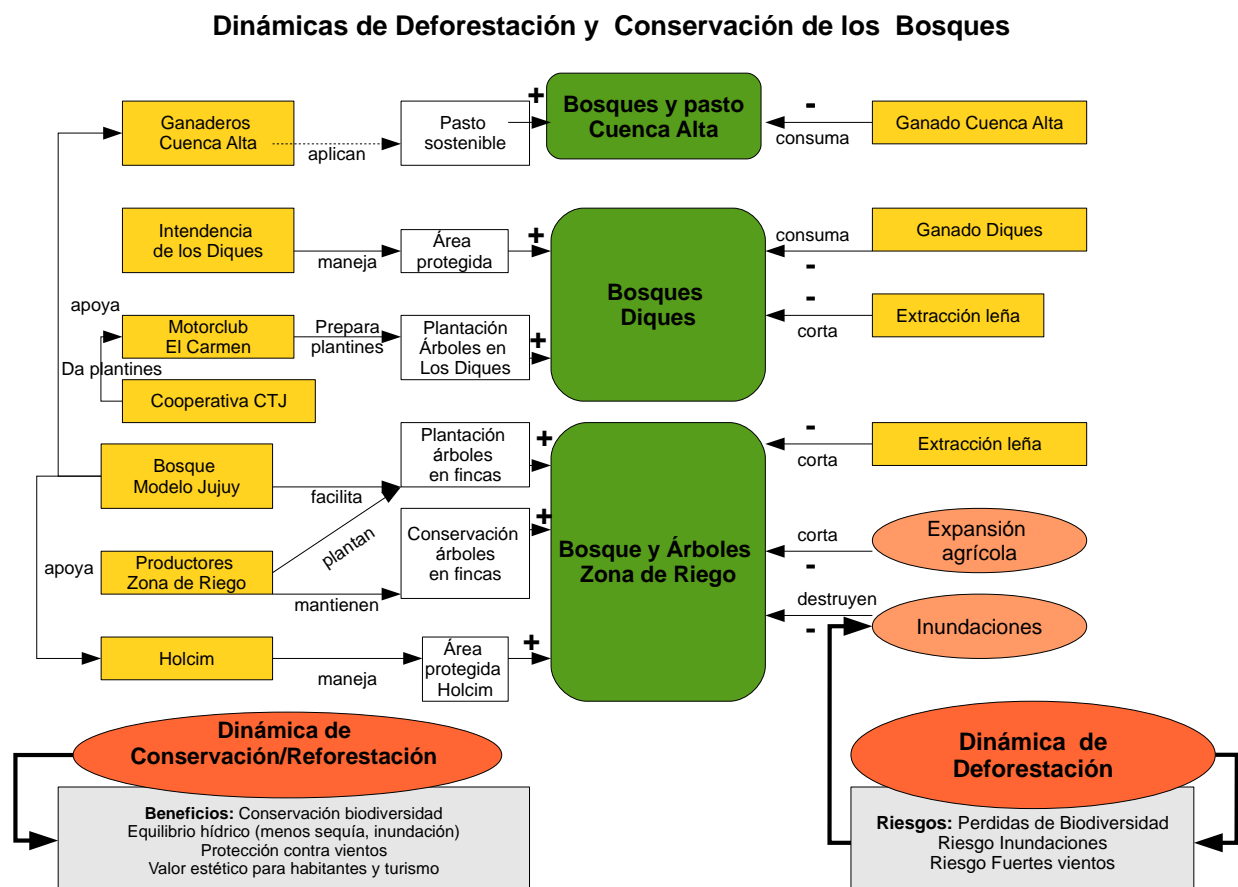
Ilustración 19: Modelo de la Deforestación y Reforestación en los Pericos-Manantiales
