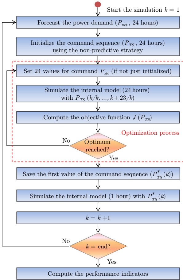
Fig. 3. MPC algorithm.
