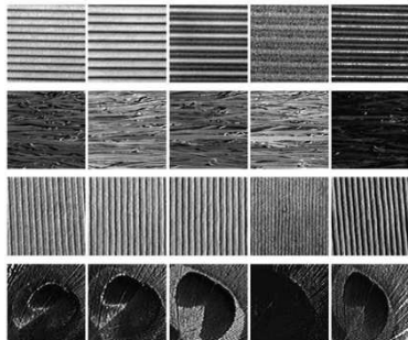
Fig. 3. CURET dataset.
