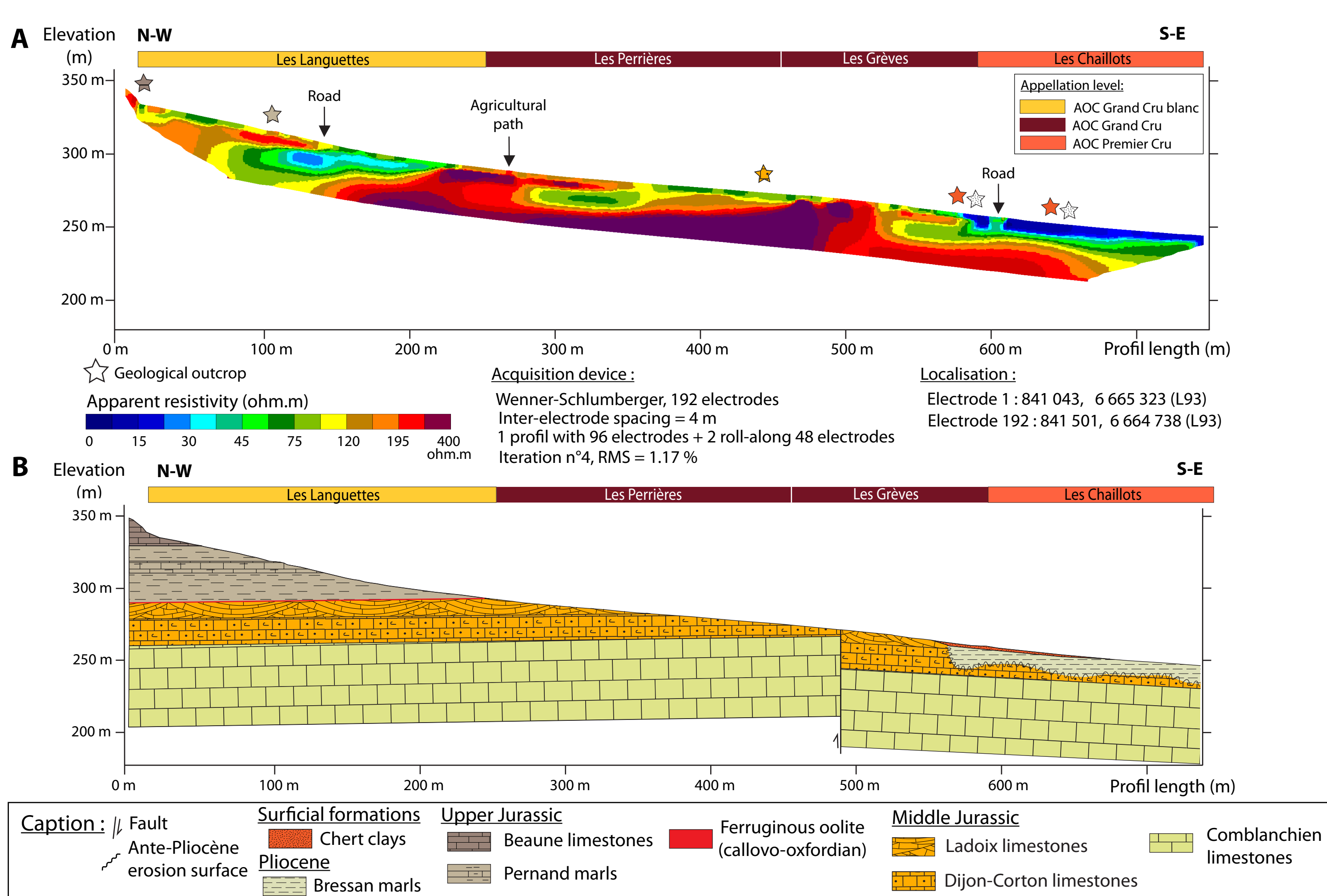
Electrical apparent resistivity profile and geological interpretation performed on the Aloxe-Corton hillslope Profil de résistivité apparente et coupe géologique interprétative réalisés sur le versant d'Aloxe-Corton
