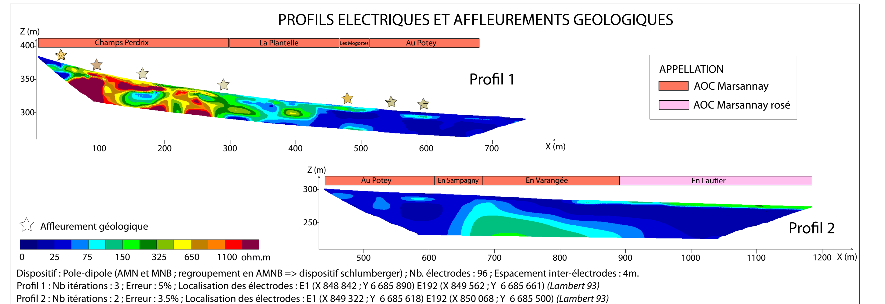
PROFILS ELECTRIQUES ET AFFLEUREMENTS GEOLOGIQUES
