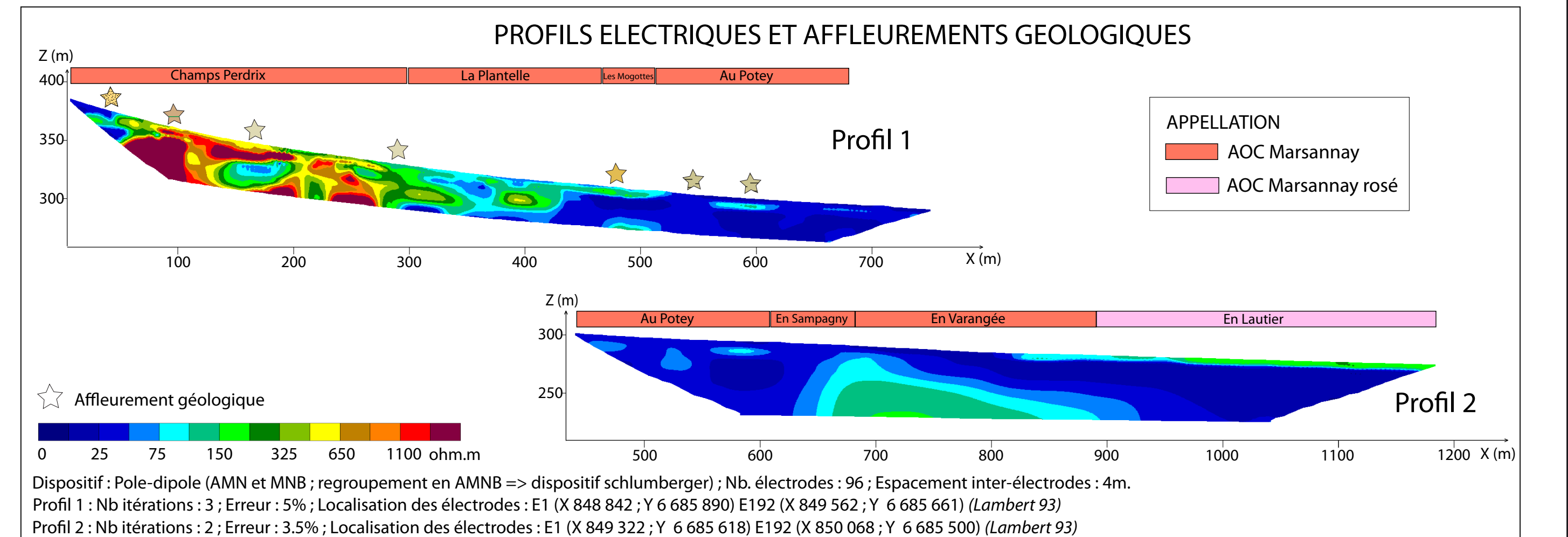
Dispositif : Pole-dipole (AMN et MNB ; regroupement en AMNB => dispositif schlumberger) ; Nb. électrodes : 96 ; Espacement inter-électrodes : 4m. Profil 1 : Nb itérations : 3 ; Erreur : 5% ; Localisation des électrodes : E1 (X 848 842 ; Y 6 685 890) E192 (X 849 562 ; Y 6 685 661) (Lambert 93) Profil 2 : Nb itérations : 2 ; Erreur : 3.5% ; Localisation des électrodes : E1 (X 849 322 ; Y 6 685 618) E192 (X 850 068 ; Y 6 685 500) (Lambert 93)
