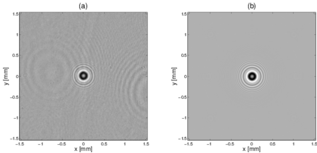
Figure 11: hologrammes d'une bulle d'air dans une goutte obtenus par (a) l'expérience, (b) la modélisation théorique
