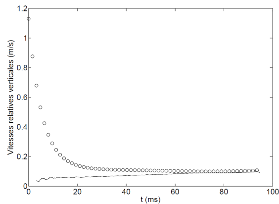
Figure 5. (o) vitesse de chute de la goutte mesurée par HN pour T^{\infty}=21,5^{\circ}\text{C} , R_h=0,70 , d_0=55,5\ \mu\text{m} , u_0=1,13\ \text{ms}^{-1} . (-) vitesse de l'air ambiant u_{\text{air}} nécessaire dans la trainée de l'équation du mouvement pour reproduire les positions, vitesses et accélérations de la goutte mesurées par HN. u_{\text{air moyen}} = 0,076\ \text{ms}^{-1} .
