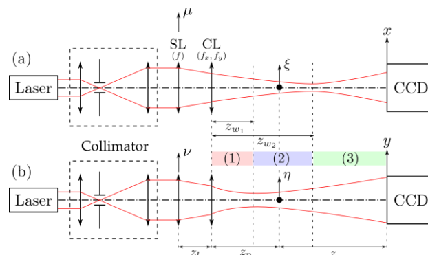
Figure 1. Dispositif expérimental pour l'enregistrement d'hologrammes avec référence astigmatique. (a) Plan x,z.
