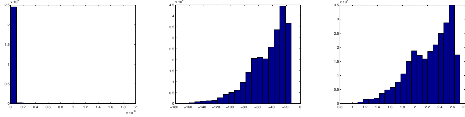
FIG. 1 – Histogramme des valeurs des matrices de Gram : noyau K_{DTW} à gauche, noyau \log(K_{DTW}) au centre et noyau K_{DTW}^t normalisé à droite.
