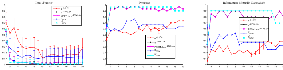
FIG. 3 – Taux d'erreur de classification 1-PPV (à gauche), précision (au centre) et information mutuelle normalisée (à gauche) pour le clustering obtenu par les K-moyennes - pour les 5 noyaux testés (Gaussien Euclidien × rouge, Gaussien DTW * noire, MCPP Gaussien DTW o rose, KDTW + bleu, KDTW t □ cyan) sur le jeu données CBF, lorsque la dimension du sous espace des caractéristiques varie de 1 à 20.
