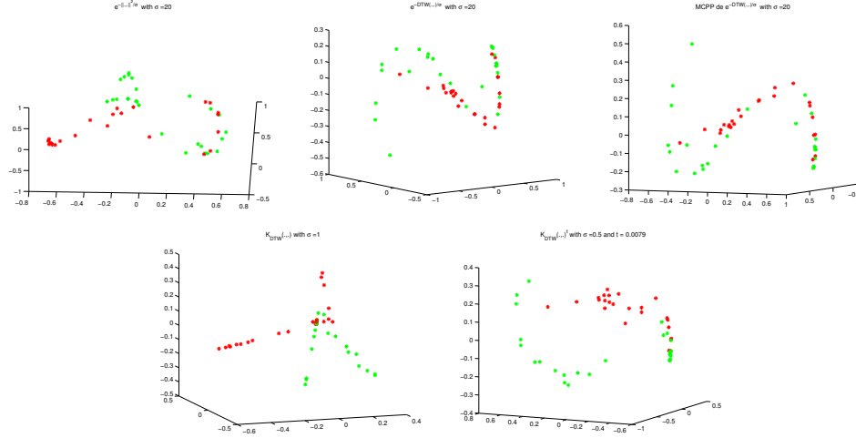
FIG. 2 – Projections des séries du jeu de données Gun_Point dans le sous espace des caractéristiques de dimension 3 obtenu par K-PCA pour les noyaux : Gaussien Euclidien (en haut à gauche), Gaussien DTW (en haut au centre), MCPP du Gaussien DTW (en haut à droite), K_{DTW} (en bas à gauche) et K_{DTW}^t (en bas à droite).
