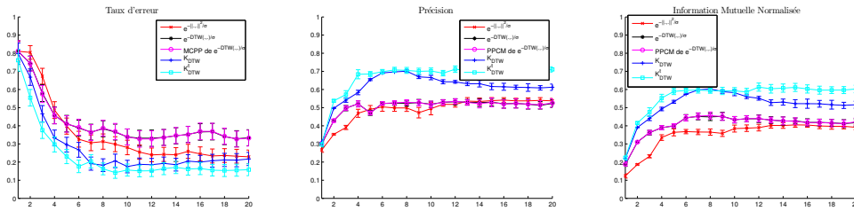
FIG. 4 – Taux d'erreur de classification 1-PPV (à gauche), précision (au centre) et information mutuelle normalisée (à gauche) pour le clustering obtenu par les K-moyennes - pour les 5 noyaux testés (Gaussien Euclidien × rouge, Gaussien DTW * noire, MCPP Gaussien DTW o rose, KDTW + bleu, KDTW t □ cyan) sur le jeu données FISH, lorsque la dimension du sous espace des caractéristiques varie de 1 à 20.
