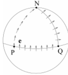
FIGURE 4.1. transport quadri-vecteur
