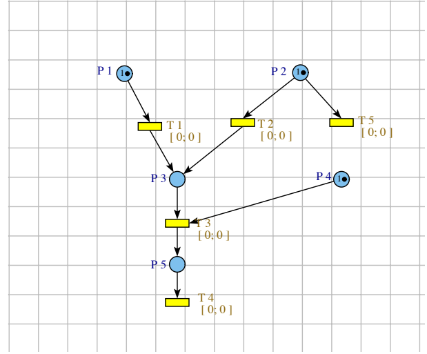
Fig. 4. Petri net
