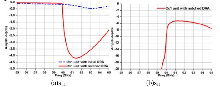
Fig. 7. S parameters for 2\times 1 unit-cell
