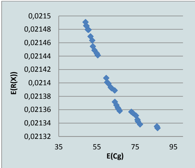
Fig. 17 Optimal Pareto front.
