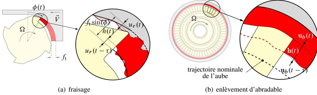
Figure 2 – Analogie entre le fraisage et l'enlèvement d'abrasable dans une turbomachine
