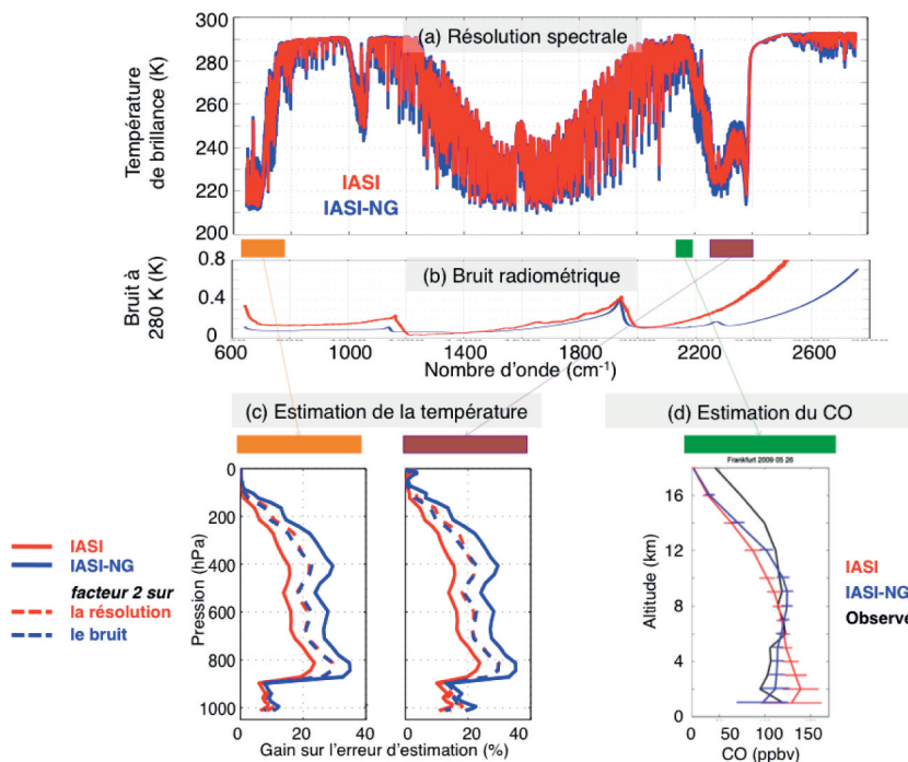
Figure 2. Caractéristiques spectrales et radiométriques de Iasi (rouge) et Iasi-NG (bleu) et leur impact sur la restitution de variables atmosphériques. (a) Spectre des températures de brillance pour une atmosphère tropicale à la résolution spectrale de Iasi et de Iasi-NG. (b) Bruits radiométriques de Iasi et Iasi-NG à une température de référence de 280 K. (c) Gain sur l'erreur d'estimation par rapport à l' a priori (%) des profils atmosphériques de température à partir de deux bandes spectrales (645-770 \text{cm}^{-1} et 2250-2420 \text{cm}^{-1} ). En pointillé, gain lorsque seule la résolution spectrale ou le bruit est amélioré. (d) Comparaison des restitutions de monoxyde de carbone (CO) à partir de Iasi et Iasi-NG et comparaison avec le vrai profil.
