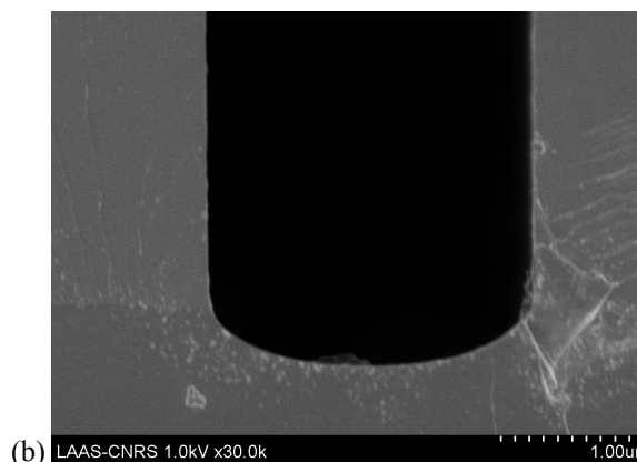
Figure 9 : Images MEB du flanc de tranchée après DRIE (a) et après oxydation de 260nm et attaque humide au buffer HF (b)
