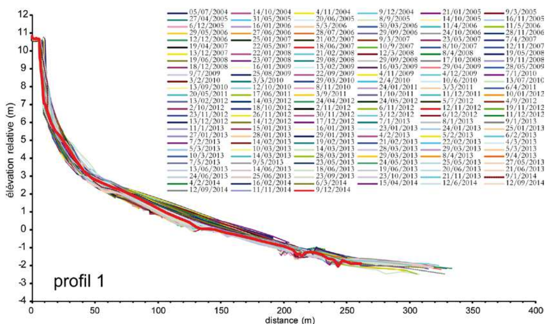
Figure 8. Exemple d'une enveloppe de profils de plage / cordon dunaire obtenue sur le profil 1 entre les mois de juillet 2004 et décembre 2014.
