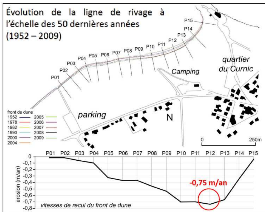
Figure 3. Evolution du trait de côte entre 1952 et 2009 au niveau de la plage de la sécherie.
