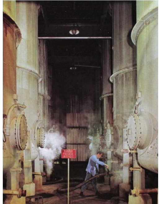
Cuves de fermentation
