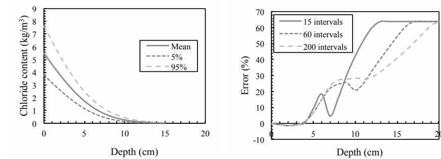
Figure 3. (a) Profils en ions chlorure à t = 10 ans - (b) Convergence du RB avec le nombre d'intervalles
