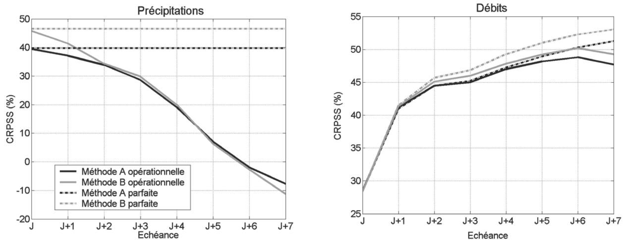
Figure 4 : Évolution du score CRPSS (%) en fonction de l'échéance pour le bassin de l'Yonne-C, lorsque les méthodes A et B de prévision par analogie sont appliquées dans les contextes de prévision parfaite et de prévision opérationnelle des précipitations.
