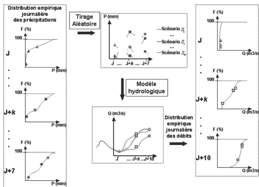
Figure 2 : Procédure schématisée de la génération de N scénarios de débits pour les échéances J à J+10 , à partir des distributions empiriques journalières des précipitations issues de la méthode d'analogie.
