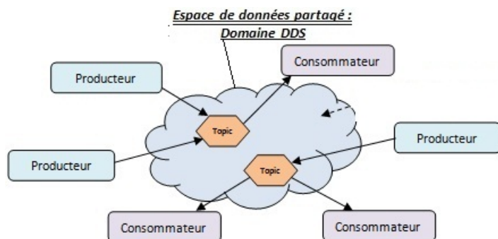
FIGURE 1: Espace de données partagé de DDS
